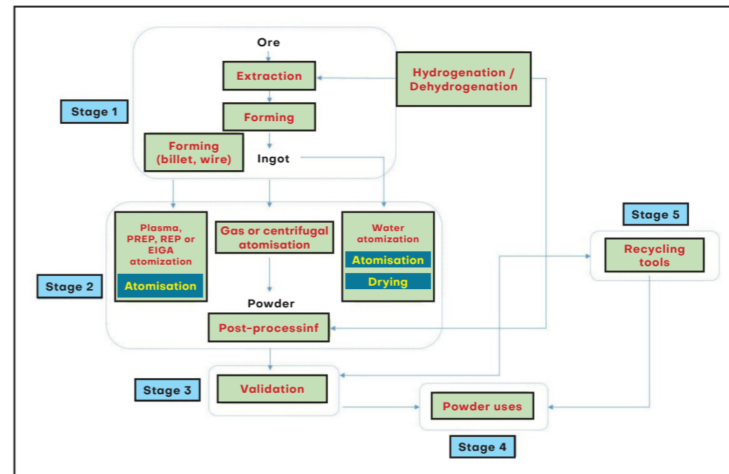
Figure : Cette figure présente un organigramme des étapes du cycle de vie de la production de poudre (adapté de Dawes et al.), où le procédé PREP-plasma rotating electrode, REP-rotating electrode process, EIGA-electrode induction melting gas atomisation) ont été exploités.
